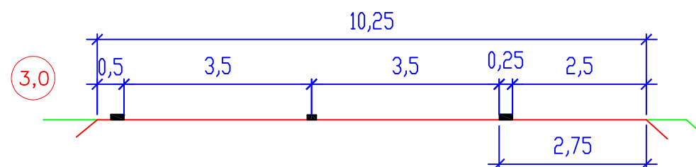
S 24,5 (ČSN 73 6101/2018)
