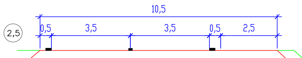
S 24,5 (ČSN 73 6101/1962)
