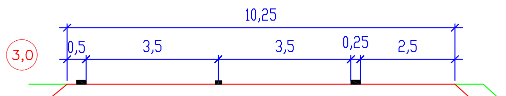
S 24,5 (ČSN 73 6101/2004)
