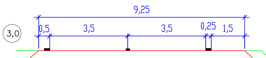
R/S 22,5 (ČSN 73 6101/1985, 2000)
