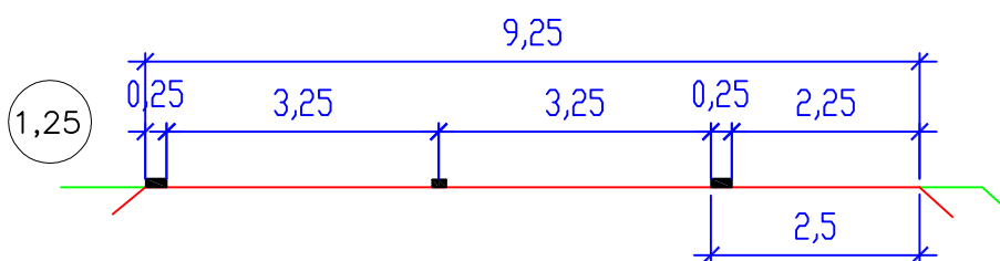
S 20,75 (ČSN 73 6101/2018)
