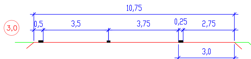
D 26,5 (Zásady 1974)
